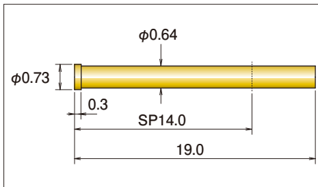
K2-0.48S-2-SP14-2 (S048-140-03)
