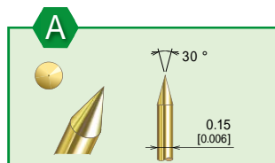
K2-0.26 III A-2M-5
